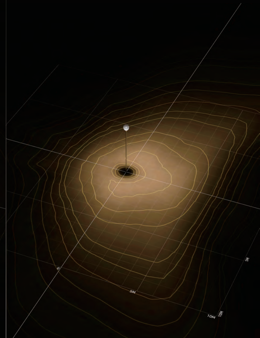
蝙蝠翼配光 BATWING
