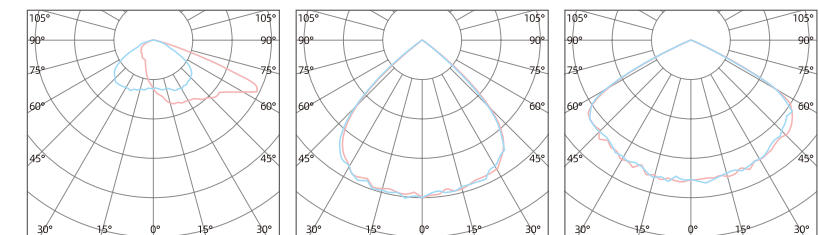
T3M 安装高度4M T3S 安装高度4M T4S1 安装高度4M
