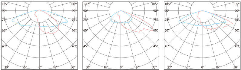
T15 安装高度4M T2M 安装高度4M T2S 安装高度4M
