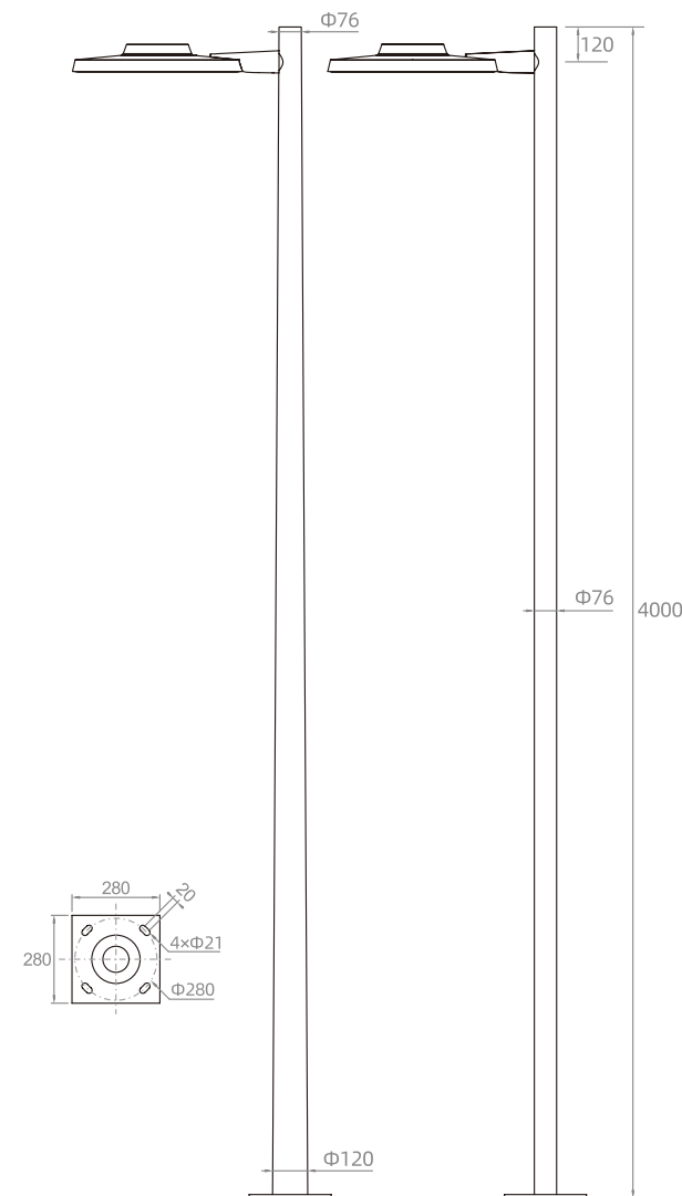
T3M 安装高度4M T3S 安装高度4M T4S1 安装高度4M
