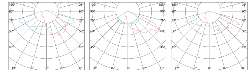
T15 安装高度4M T2M 安装高度4M T2S 安装高度4M
