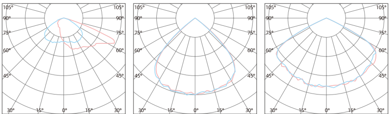
T3M 安装高度4M T3S 安装高度4M T4S1 安装高度4M
