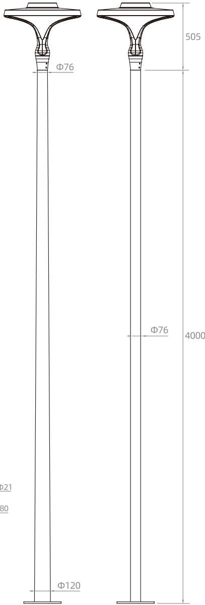
T15 安装高度4M T2M 安装高度4M T2S 安装高度4M
