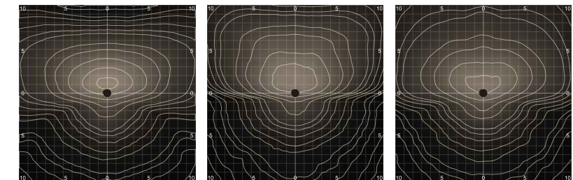
T3M 安装高度4M T3S 安装高度4M T4S1 安装高度4M
