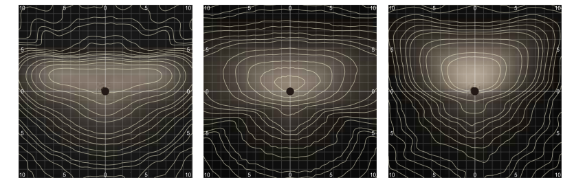
T15 安装高度4M T2M 安装高度4M T2S 安装高度4M
