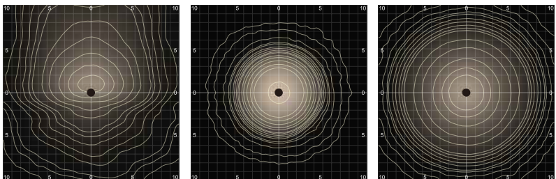
T4S2 安装高度4M 90° 安装高度4M 120° 安装高度4M
